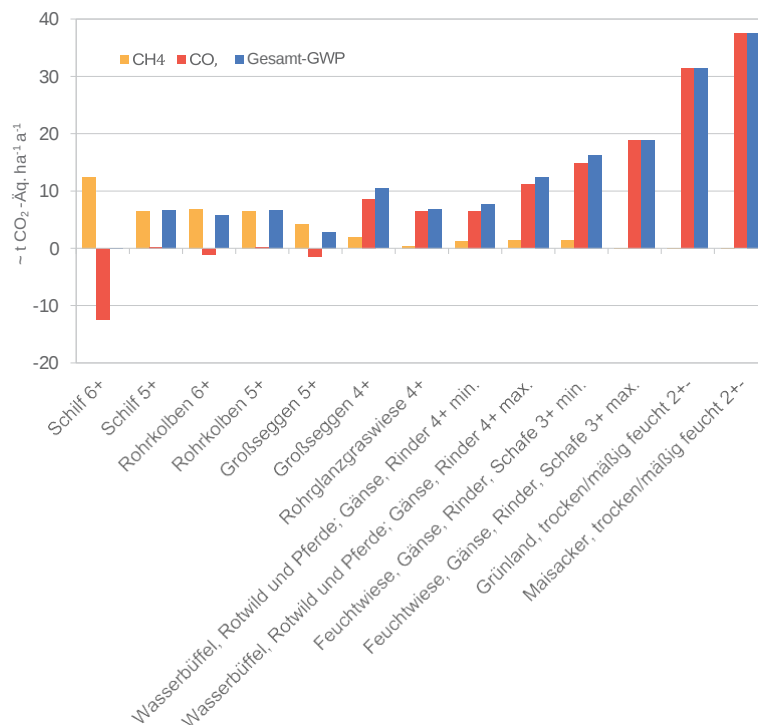
Abbildung 4.3: Übersicht der geschätzten Standortemissionen der in KLIBB betrachteten Bewirtschaftungsverfahren. Voraussichtlich langfristige Treibhausgas-Emissionen ausgedrückt als Global Warming Potential (GWP). Aus: Närmann et al. (2021, S. 143)
