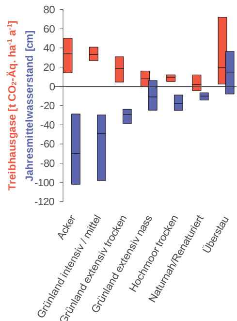
Abbildung 4.2: Mittelwert, Minimum und Maximum der gemessenen Jahresmittelwasserstände (vgl. Tab. 4.2 ) in blau und jährliche Treibhausgasbilanzen in rot nach Nutzungskategorien.
