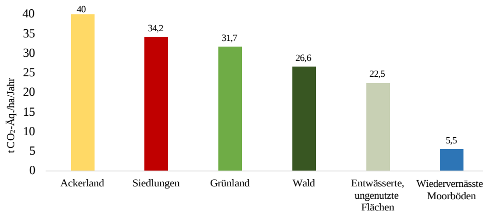
Abbildung 3.5: Treibhausgas-Emissionen in Deutschland nach Landnutzungstyp. Daten aus Tiemeyer et al. (2020)
