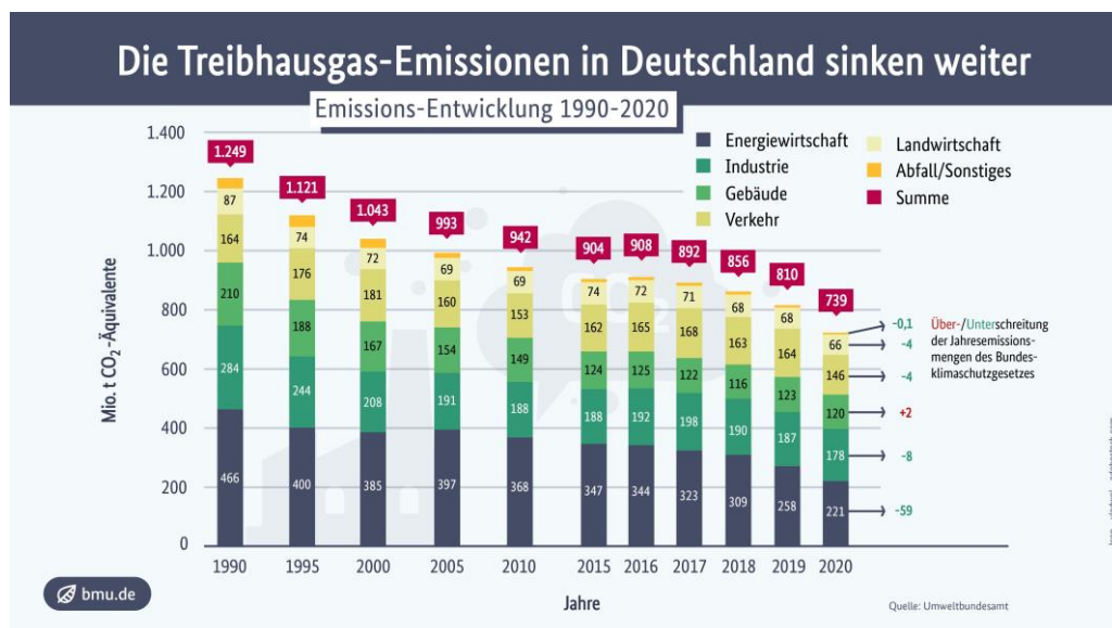
Abbildung 3.3: Das Balkendiagramm zeigt die Entwicklung der gesamten Treibhausgasemissionen nach Sektoren von 1990 bis 2020. Es ist ein Abwärtstrend zu verzeichnen: Im Zeitraum von 1990 bis 2020 sind die Treibhausgasemissionen von knapp 1,25 Mrd. auf 739 Mio. t CO 2 -Äquivalente gesunken. Übernommen aus: BMUV (2022)
